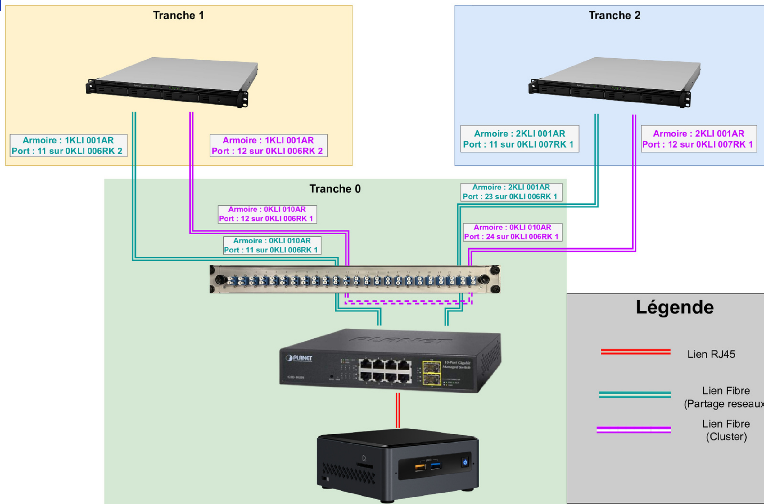
Schema Resaux NAS
